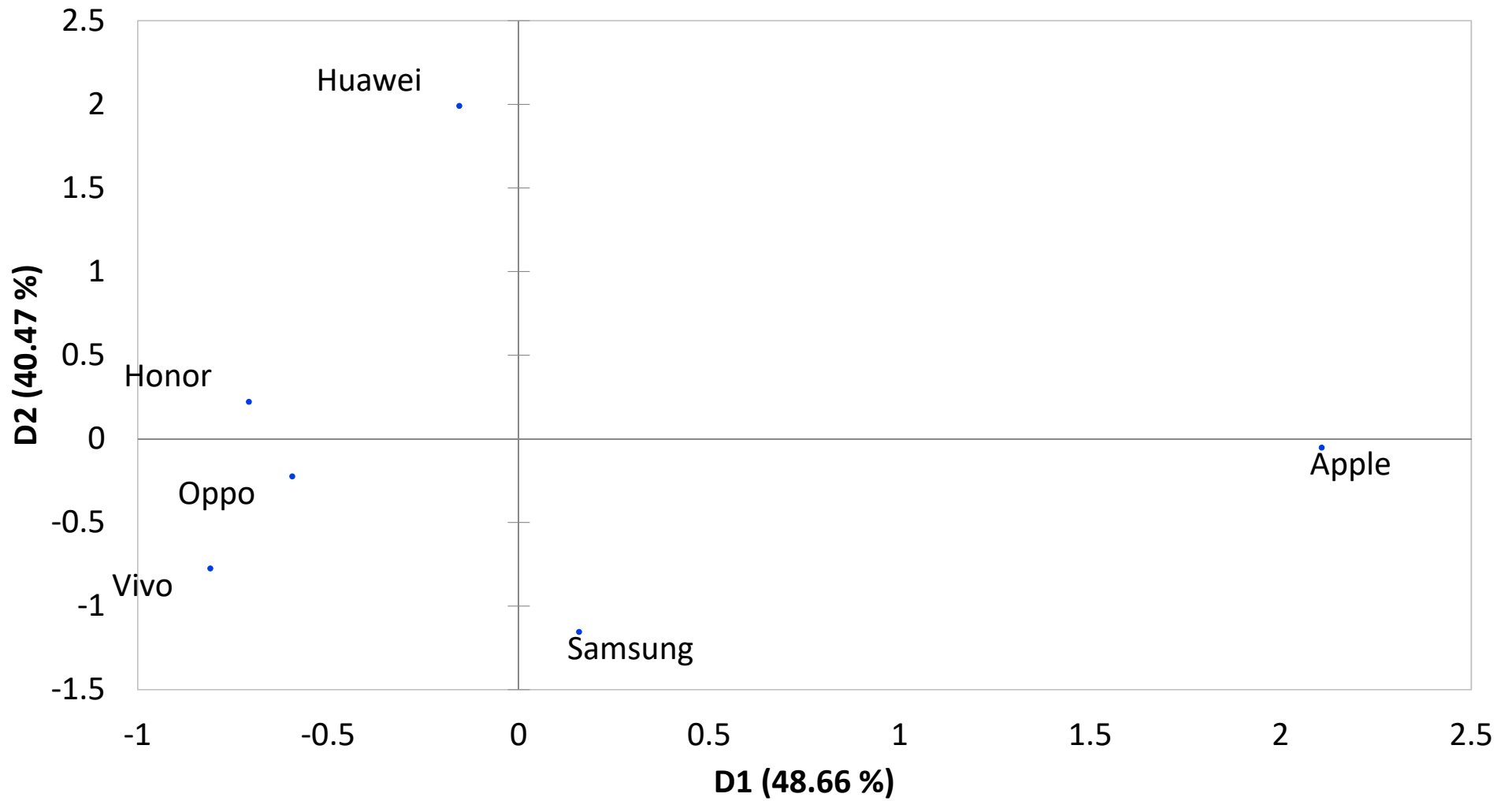
Observations (axes D1 and D2: 89.13 %)
