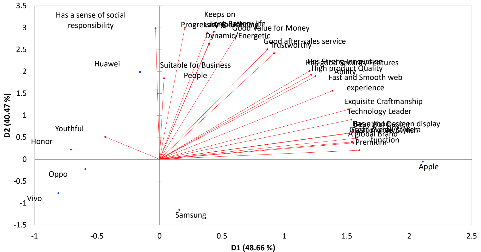
Biplot (axes D1 and D2: 89.13 %)
